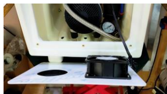
Ventilateur de refroidissement sur plaque amovible.
